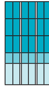
Layout 2 5 Ebenen, 28 Wahlen z. B. 3 Ebenen PET 0,5 l (162) 1 Ebene Dose 0,33 l (54) 1 Ebene PET 1,0 l (28)
